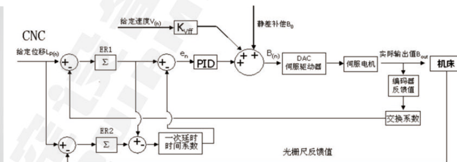
双位置闭环
